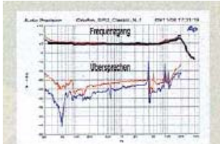
Ortophon SPU Classic: bis 20 kHz vorbildlich linear; etwas stärkeres, aber symmetrisches Übersprechen.
