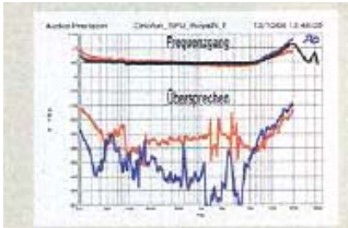
Ortophon SPU Royal: schon merklicher Hochtonanstieg; Übersprechen nicht ganz symmetrisch.
