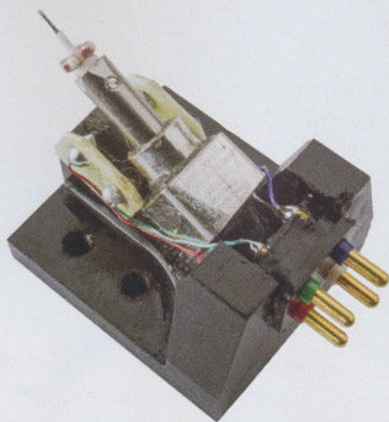
Für alle Gegebenheiten hat das System zwei Paar eingeschnittene Gewinde zur Montage
