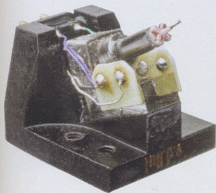
Durch den Verzicht auf das vordere Joch muss der verbleibende Magnet umso kräftiger sein, um die hohe Ausgangsspannung zu erreichen
